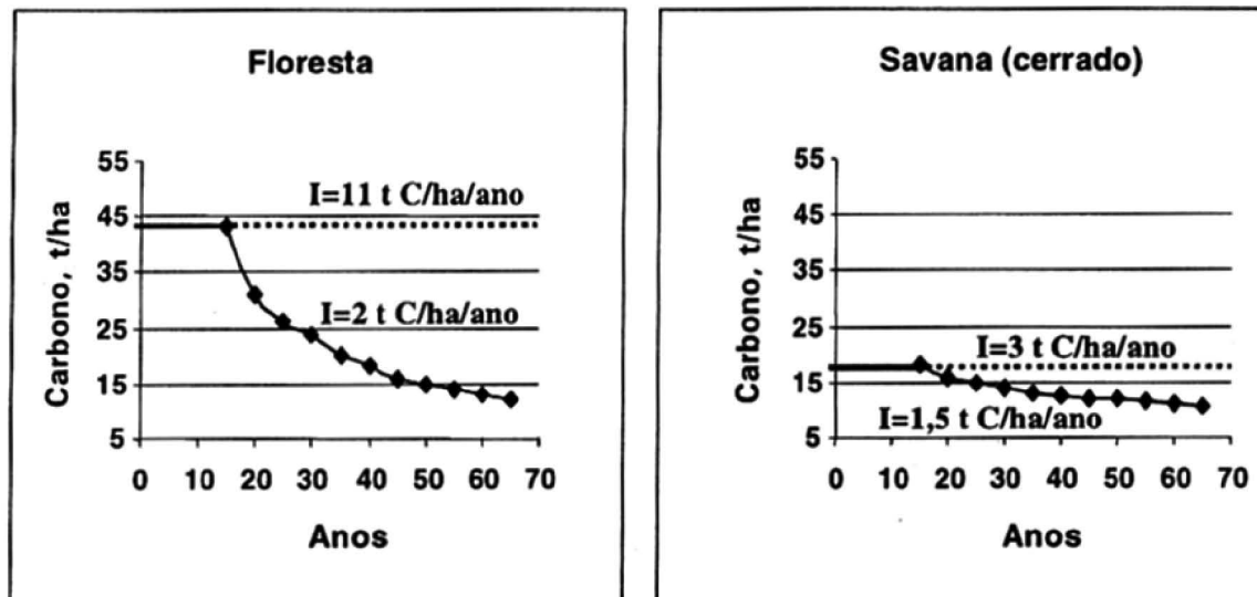
FIGURA 3. Simulação dos efeitos de desmatamento e cultivo sobre o estoque de carbono em dois ecossistemas tropicais, floresta e cerrado. I = 'Input' de C por ha/ano. Fonte: Adaptado de Scholes et al. (1997) e Jenkinson (1990).
