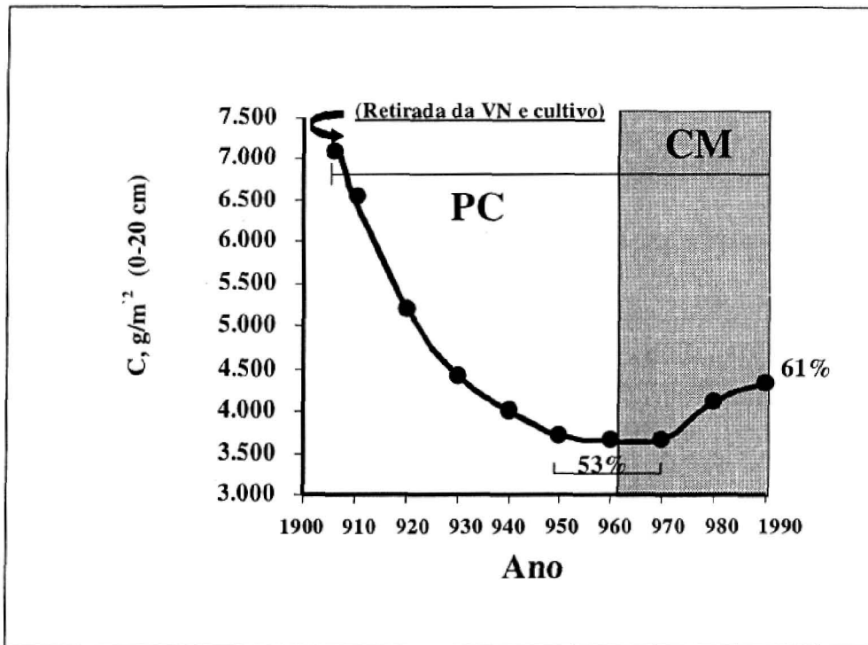
FIGURA 4. Estoque de carbono em solo (0-20 cm) de região temperada sob efeito de retirada da vegetação natural, VN, cultivo e de sistemas de preparo do solo. I = 'input' de C por ha/ ano, PC, plantio convencional; CM, cultivo mínimo. Fonte: adaptado de Donigian al (1994)
