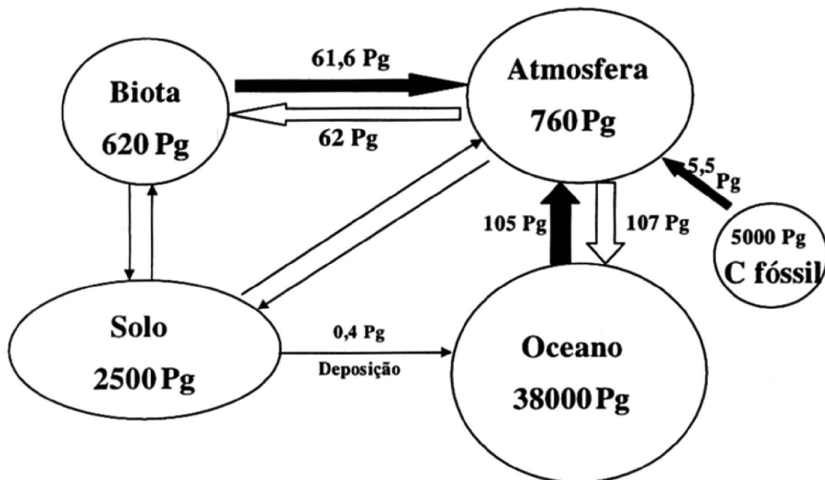
FIGURA 1. Ciclo e compartimentos globais do carbono. Fonte: Lal (1999).
