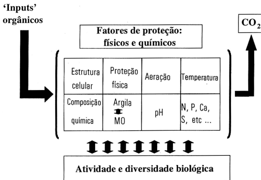
FIGURA 2. Fatores que condicionam a decomposição de resíduos orgânicos no solo. Fonte: Noordwijk et al. (1997).
