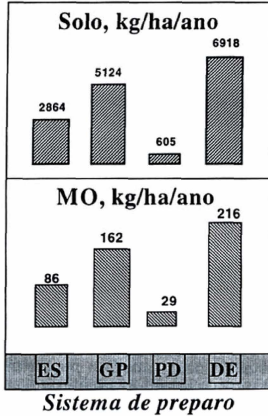
FIGURA 5. Perdas médias de solo e matéria orgânica (MO) sob influência de sistemas de preparo do solo. ES: escarificação + gradagem niveladora; GP: gradagens (pesada + niveladora); PD: plantio direto; DE: aração com discos + duas gradagens niveladoras. Fonte: Hernani et al. (1999).
